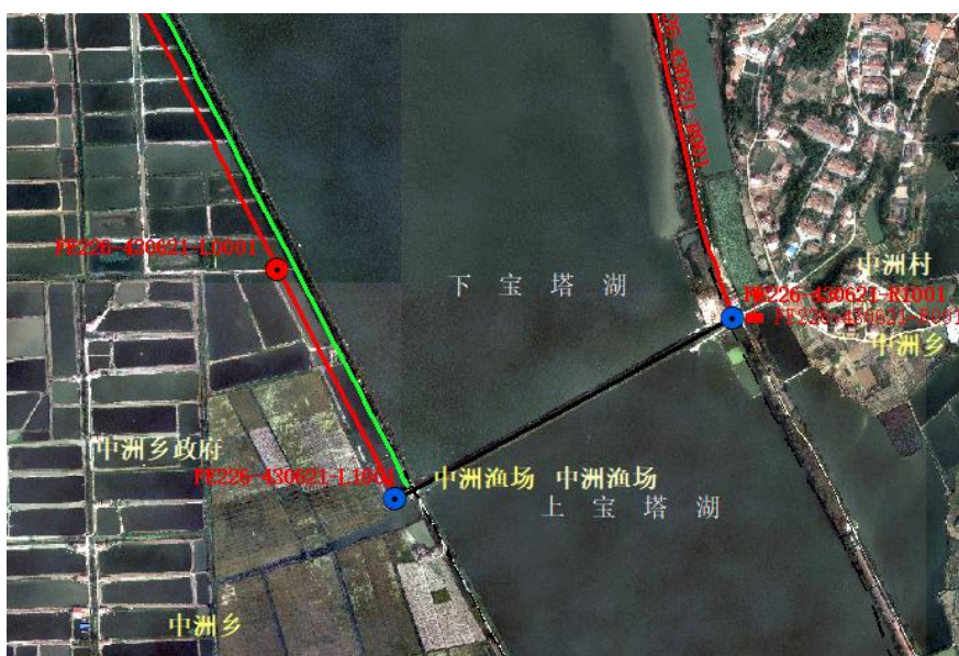
图 4.3-2 下宝塔湖湖湖交界处公共桩示意图
