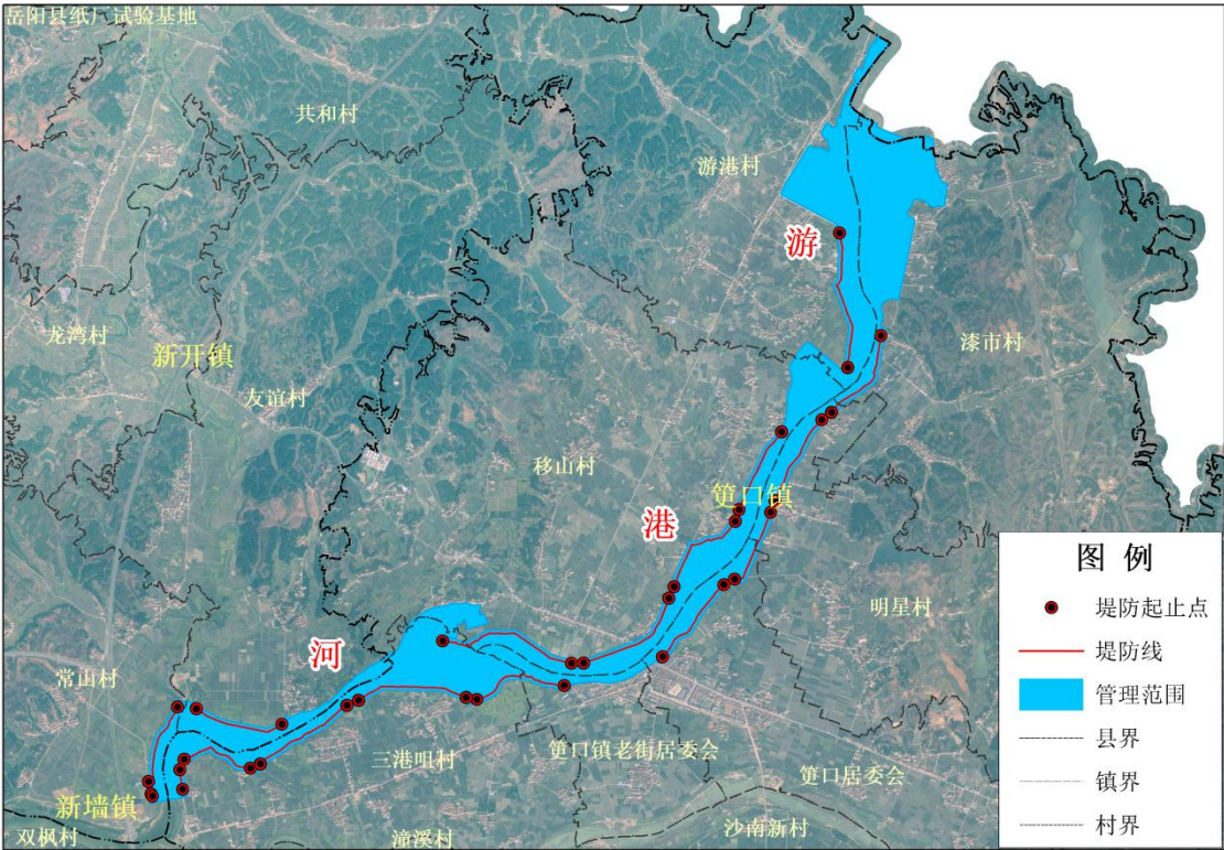
图 2.2-1 游港河岳阳县管理范围简图
